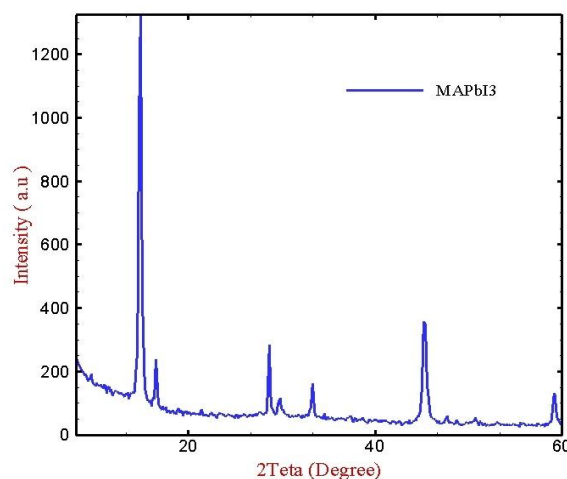
شکل ۲: طیف XRD از MAPbI_3
