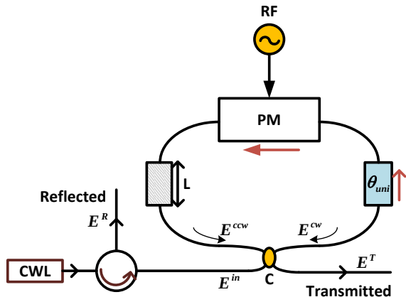
شکل ۱. تداخل سنج ساگناک شامل تحریرگر فاز و محیط دارای رفتار
