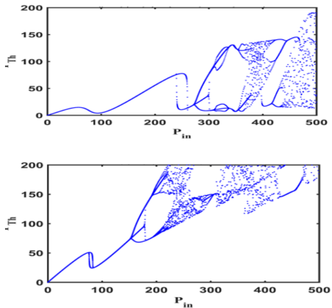
شکل ۳) نمودار شدت خروجی بر حسب شدت میدان از مشدد حلقوی دارای جفتگر الف) همسان \beta_1 = \beta_2 ب) ناهمسان به ازای \beta_1 = 1; \beta_2 = 3
