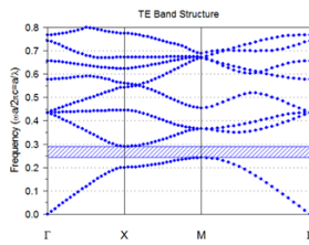
(ب) شکاف باند فوتونی مربوط به (الف)
