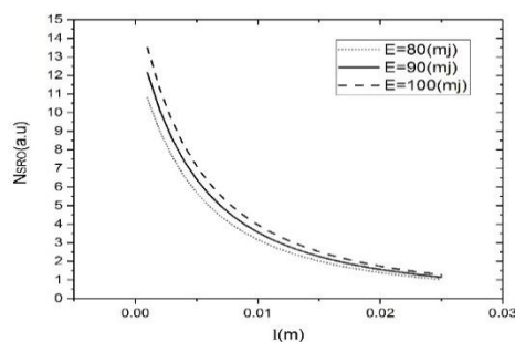
شکل ۵: طول بلور BBO برحسب N_{SRO} در تقریب موج تخت.
