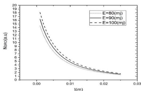
شکل ۶: طول بلور BBO برحسب N_{SRO} در تقریب موج تخت
