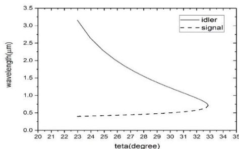
شکل ۴: زاویه‌های تطبیق فاز نوع (ooe) نسبت به طول موج های سیگنال و ایدلر برای طول موج پمپ ۳۵۵ نانومتر
