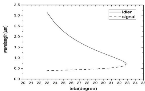
شکل ۱: زاویه‌های تطبیق فاز نوع (ooe) نسبت به طول موج های سیگنال و ایدلر برای طول موج پمپ ۳۵۵ نانومتر
