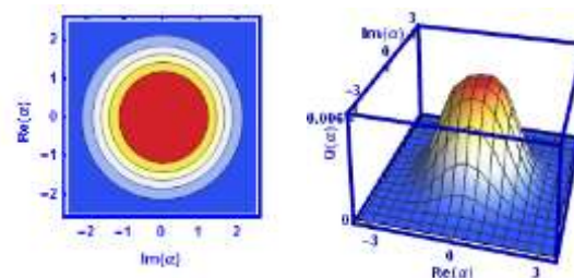
شکل ۳: تابع توزیع هوسیمی و نمودار کنتور متناظر با آن به ازای \lambda=3 و \zeta=0.5 ، \bar{n}=50 ، \alpha=x+iy
