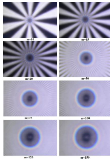
شکل ۲: طرح های پراش برای توری های شعاعی رانکی با تعداد پره های مختلف. توری ها در فاصله Z=80 سانتی از دوربین قرار گرفته اند. با بالا رفتن تعداد پره‌ها، شعاع حلقه‌های رنگی طبق رابطه ۴ افزایش پیدا می‌کنند.
