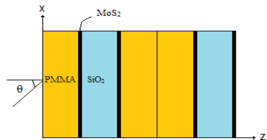
شکل ۴: طرح شماتیک ساختار یک بعدی شبه پریودیک فیبوناچی مرتبه چهارم شامل تک لایه های \text{MoS}_2 .
