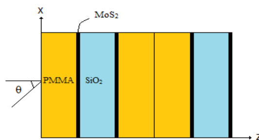
شکل ۴: طرح شماتیک ساختار یک بعدی شبه پریودیک فیبوناچی مرتبه چهارم شامل تک لایه های \text{MoS}_2 .
