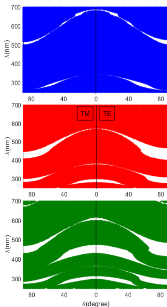
شکل ۴: ساختار باند بلور فوتونی شبه پریودیک فیبوناچی برحسب زاویه تابش و طول موج برای مرتبه ۳ (آبی)، مرتبه ۴ (قرمز) و مرتبه ۵ (سبز) برای دو قطبش TE و TM.
