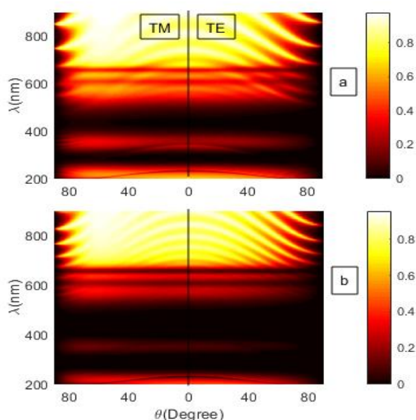
شکل ۳: تراگسیل بلور فوتونی شبه پریودیک فیبوناچی بر حسب زاویه تابش و طول موج برای مرتبه ۳ (a) و مرتبه ۴ (b) برای دو قطبش TE و TM.
