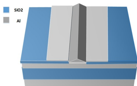
شکل ۱- الف: سلول واحد ساختار حسگر
