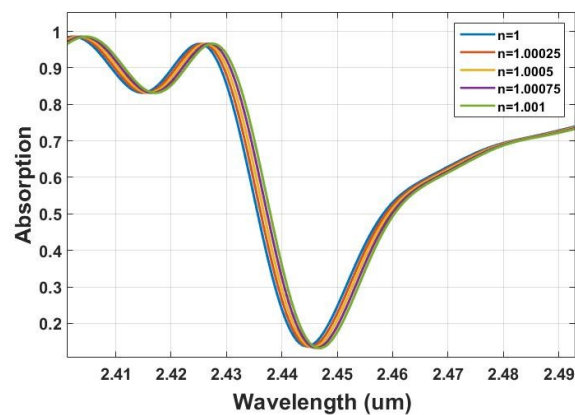
شکل ۴-ب: طیف بازتاب بر حسب تغییرات ضریب شکست به اندازه 10^{-3}
