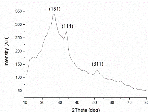
شکل ۱) نمودار پراش اشعه ایکس نانو کامپوزیت پلی متیل متاکریلات-پلی آنیلین-سولفیدقلع
