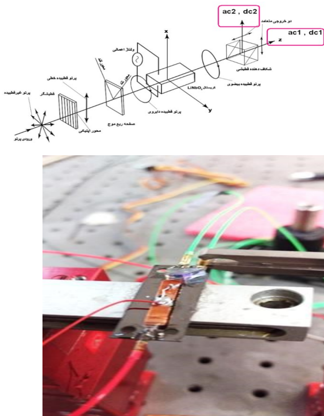
شکل ۱: ساختار حسگر نوری ولتاژ دو خروجی برپایه نگه‌دارنده سیلیکون
