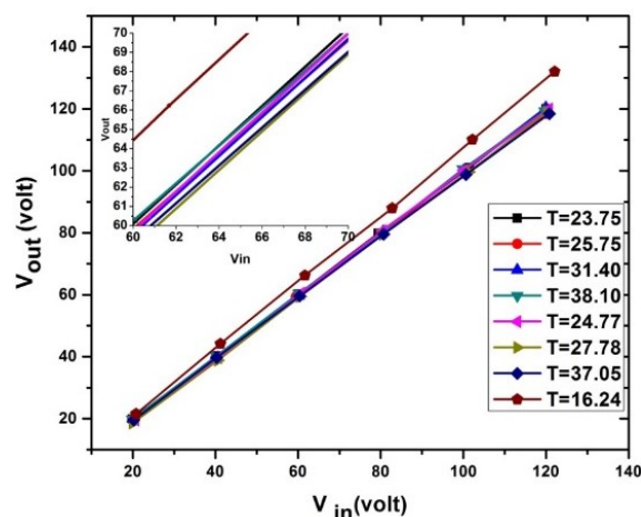
شکل ۶: بررسی خطی بودن خروجی حسگر
