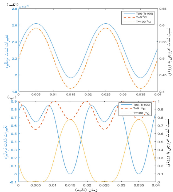
شکل ۳: شکل موج تغییرات دمایی خروجی سنسور در دو دمای صفر و 100^\circ\text{C} درجه سانتی‌گراد و تفاضل این دو: (الف) برش X و انتشار در راستای Z (ب) برش Z و انتشار در راستای Y
