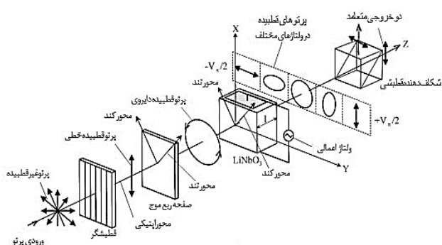
شکل ۱: ساختار شماتیک سنسور اپتیکی ولتاژ
