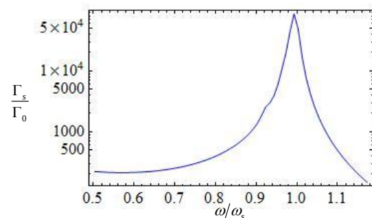
شکل ۱: آهنگ گسیل خودبه‌خودی بدون بعد \Gamma_s/\Gamma_0 برحسب بسامد بدون بعد \omega/\omega_s . در این‌جا \Gamma_0 آهنگ گسیل خودبه‌خودی اتم مزبور در خلأ است.
