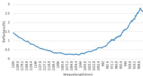
شکل ۲: منحنی طیف بازتابی اندازه گیری شده نمونه
