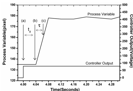
شکل ۲: پاسخ زمانی سیستم کنترل به سیگنال اعمال شده. در این نمودار t_d تاخیر بین لحظه اعمال ولتاژ به سیستم کنترل و لحظه شروع به حرکت نوارهای تداخلی است و \tau مدت زمانی است که طول می‌کشد تا جابه‌جایی نوارهای تداخلی به ۶۳٪ بیشینه خود برسد.
