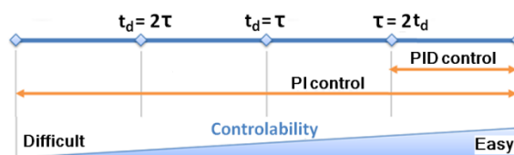
شکل ۳: ارتباط بین نسبت زمانهای تاخیر t_d با نوع سیستم کنترلی مورد استفاده.
