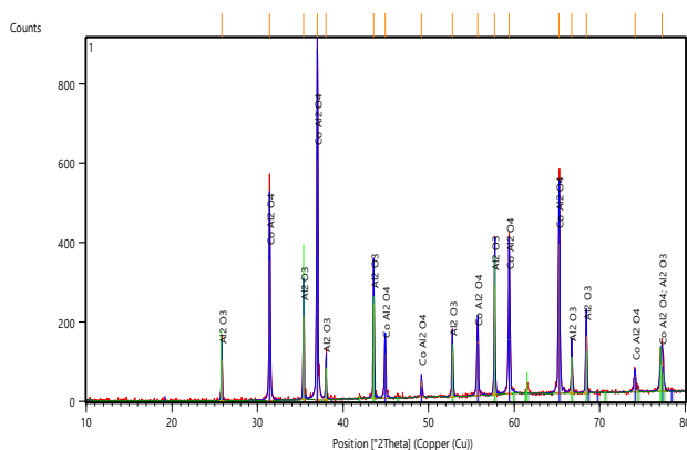
شکل ۲: طیف پراش پرتو X رنگدانه \text{CoAl}_2\text{O}_4
