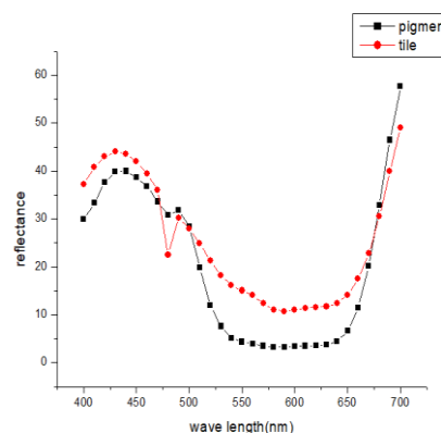
شکل ۴: طیف بازتاب مربوط به رنگدانه ساخته‌شده و چاپ آن بر روی کاشی
