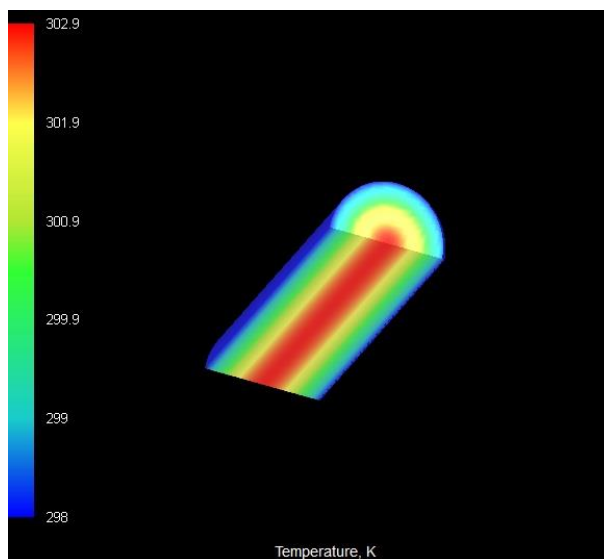
شکل ۴: توزیع حرارتی محیط فعال مایع حاوی نانو ذرات Nd_2O_3 پراکنده شده در دی متیل سولفو کسید d_6 با نرم افزار LASCAD
