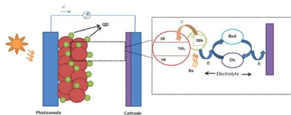
شکل ۱: طرح شماتیک سلول خورشیدی ساخته شده [۱]
