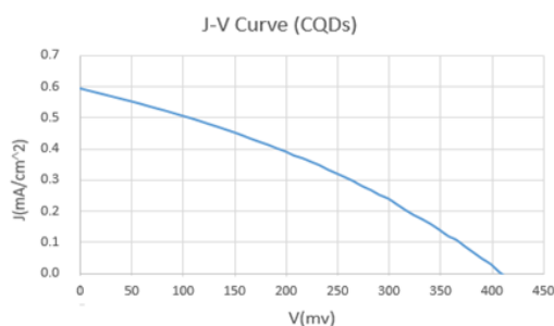
شکل ۴: منحنی چگالی جریان-ولتاژ مربوط به سلول خورشیدی حساس شده به CQDs سنتز شده
