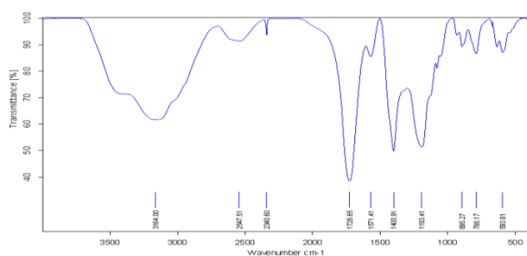
شکل ۳: نمودار FTIR مربوط به N-CQDs سنتز شده
