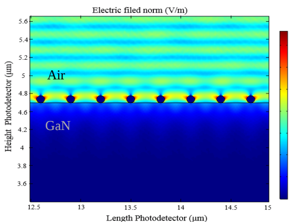
شکل ۵. اندازه میدان الکتریکی آشکارساز پلاسمونی.
