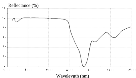
شکل ۲: طیف بالا مربوط به آینه ۳-۵ میکرومتر ساخته شده نهایی می‌باشد. محور افقی برحسب طول موج و محور عمودی، درصد انعکاس را نمایش می‌دهد. این طیف انعکاس نسبی، با استفاده از دستگاه FTIR و نسبت به طلا در زاویه ۱۲ درجه گرفته شده است.
