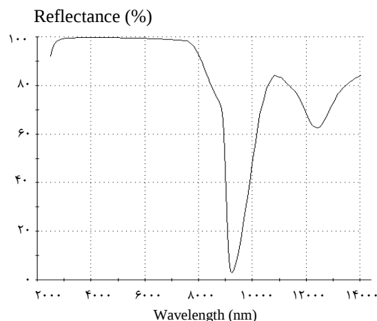
شکل ۱: منحنی بازتاب آینه‌ی کامل ۳-۵ میکرومتر. افت شدید انعکاس در بازه‌ی طول موجی ۹۰۰۰ نانومتر به اثرات جذبی \text{SiO}_2 مربوط می‌باشد. طراحی و شبیه‌سازی توسط نرم افزار طراحی لایه‌های نازک انجام شد.
