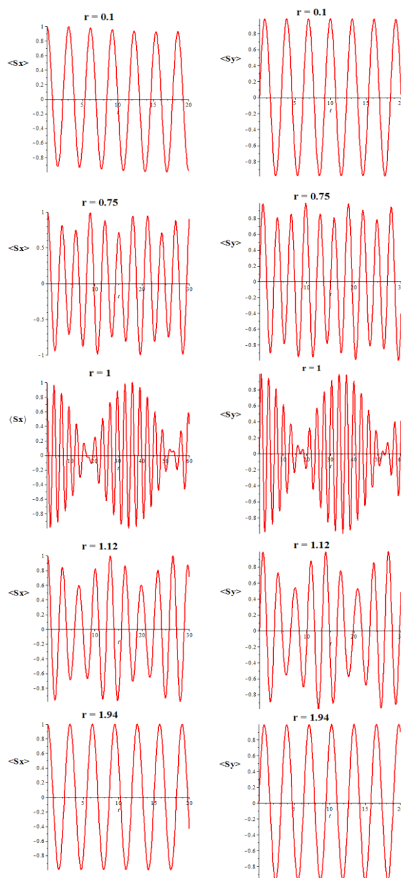
شکل ۲: تغییرات مؤلفه‌های اسپینی بر حسب زمان، به ازای s = 0.01 ، برای چند پارامتر کمناش مختلف (محور افقی بر حسب \frac{\lambda_{SO}}{\hbar} مقیاس بندی شده است).
