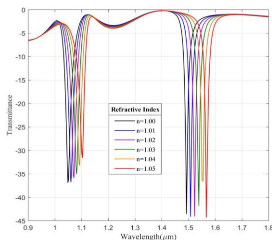
شکل ۳: منحنی عبور ساختار پیشنهادی به ازای تغییرات ضریب شکست
