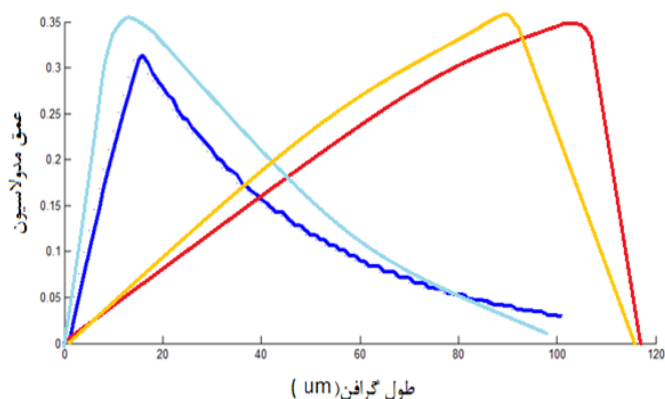
شکل ۴- عمق مدولاسیون در دو شعاع ۰/۴ و ۱ میکرومتر با و بدون روکش پلیمری در طول های مختلف گرافن
