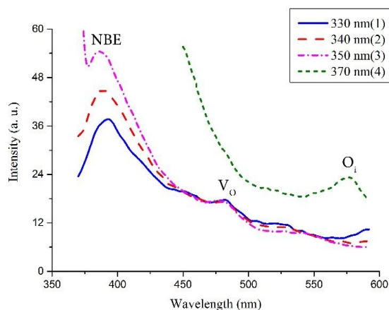
شکل ۳. طیف‌های فوتولومینسانس نانوسیم‌های ZnO که توسط طول موج‌های متفاوتی برانگیخته شده‌اند. (۱) ۳۳۰ nm، (۲) ۳۴۰ nm، (۳) ۳۵۰ nm، (۴) ۳۷۰ nm.
