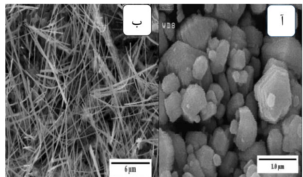
شکل ۲. تصویر SEM از لایه‌ی نازک روی (آ) پیش و (ب) پس از اکسیداسیون به مدت ۱ ساعت در دمای ۵۰۰ °C با شارش اکسیژن ۴۰ sccm.
