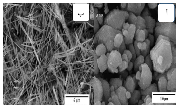
شکل ۲. تصویر SEM از لایه‌ی نازک روی (آ) پیش و (ب) پس از اکسیداسیون به مدت ۱ ساعت در دمای ۵۰۰ °C با شارش اکسیژن ۴۰ sccm.
