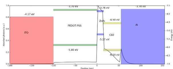
شکل ۷- نمودار جذب فوتون در تمامی لایه‌های دستگاه B
