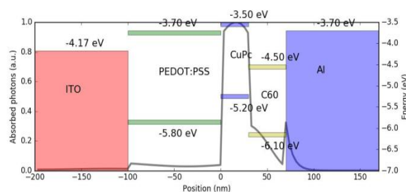
شکل ۶- نمودار جذب فوتون در تمامی لایه‌های دستگاه A
