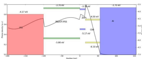
شکل ۵- نمودار تراکم فوتون در تمامی لایه‌های دستگاه B
