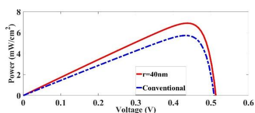
شکل ۷: منحنی توان - ولتاژ سلول خورشیدی
