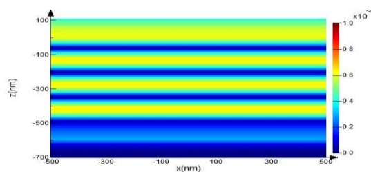
شکل ۳: میدان مغناطیسی در سلول خورشیدی حالت پایه
