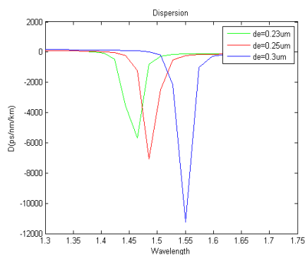
شکل ۴. پاشیدگی برحسب طول موج را به ازای مقادیر مختلف d_e برای d_2=0.46\mu m, d_1=0.96\mu m, \Lambda=1.26\mu m
