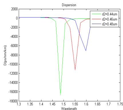
شکل ۵. تاثیر تغییرات قطر حفره‌های هوای حلقه سوم، d_2 را بر مقدار پاشیدگی منفی و \lambda_p به ازای \Lambda=1.26\mu m, d_1=0.96\mu m و d_e=0.3\mu m
