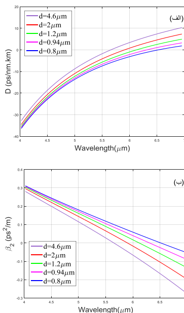
شکل ۲: (الف) مقایسه پروفایل پاشندگی برای قطرهای مختلف حفره. (ب) مقایسه ضریب پاشندگی مرتبه دوم برای قطرهای حفره متفاوت.
