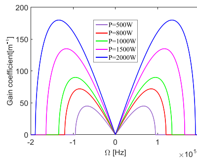
شکل ۵: ضریب بهره بر حسب واکوکی فرکانسی برای توان‌های قله پمپ متفاوت.
