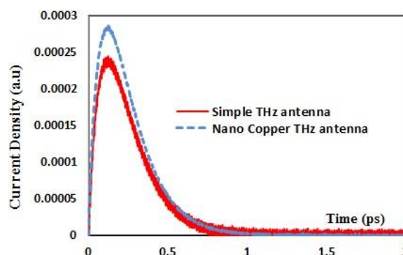
شکل ۳- چگالی جریان نوری در ناحیه گپ آنتن
