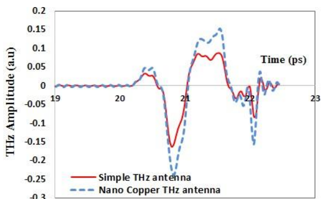
شکل ۵- نمودار زمانی پالس تراهرتز ساطع شده از آنتن
