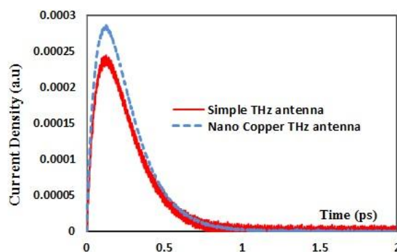
شکل ۳- چگالی جریان نوری در ناحیه گپ آنتن
