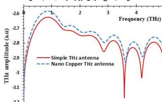
شکل ۴- طیف پالس تراهرتز ساطع شده از آنتن
