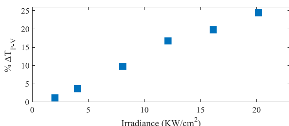
شکل ۷: نمودار فاصله قله-دره منحنی روزنه بسته جاروب Z بر حسب شدت پرتو ورودی.
