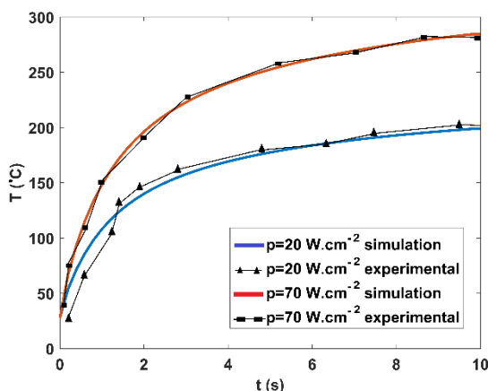
شکل ۱: تغییرات دما در مرکز برهمکنش به صورت تجربی و شبیه سازی
