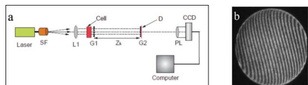
شکل ۱. طرحواره ای از انحراف سنجی ماره ای، شامل سلول حاوی سیال و توری های رانگی G_1 و G_2 و پرده
