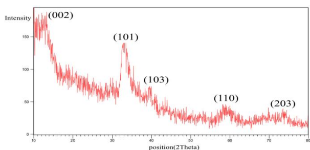
شکل ۲: طیف XRD لایه نازک WS_2 با ضخامت ۱۹۰ نانومتر
