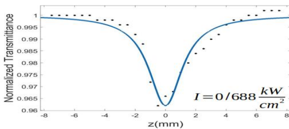
شکل ۵: نمودار پویش Z روزنه باز برای لایه نازک WS_2 با ضخامت ۱۹۰ نانومتر در دو شدت متفاوت
