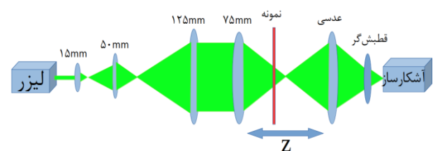
شکل ۳: چیدمان پویش Z لیزر پیوسته با طول موج ۵۳۲ نانومتر
