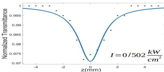
شکل ۴: نمودار پویش Z روزنه باز برای لایه نازک WS_2 با ضخامت ۳۰ نانومتر در دو شدت متفاوت
