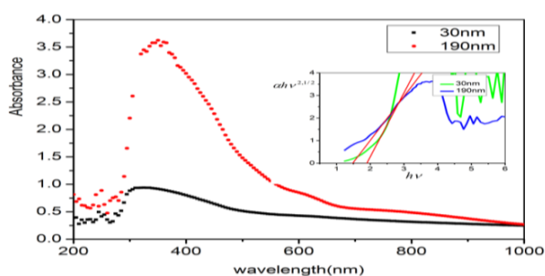
شکل ۱: نمودار جذب و نمودار تائوک مربوط به لایه‌های نازک WS_2 با ضخامت ۳۰ و ۱۹۰ نانومتر
