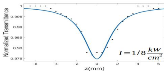
شکل ۴: نمودار پویش Z روزنه باز برای لایه نازک WS_2 با ضخامت ۳۰ نانومتر در دو شدت متفاوت
