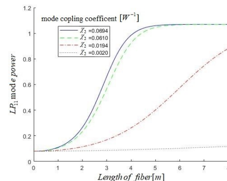
شکل ۳: تاثیر ضریب جفت شدگی مدی بر توان نرمال شده مد مرتبه بالاتر در امتداد محور اصلی فیبر.
