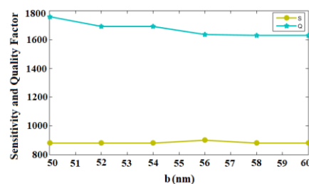
شکل ۴: بهینه‌سازی ضلع پایین دوزنقه و محاسبه حساسیت (نمودار سبز-دایره) و کیفیت (نمودار آبی-ستاره) حسگر پیشنهادی.
