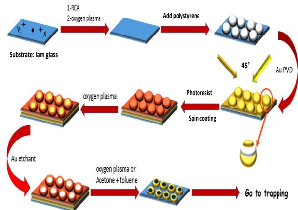
شکل ۱: شمای کلی فرآیند ساخت
