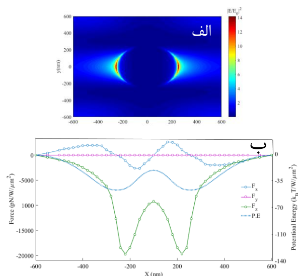
شکل ۴: شبیه سازی به دام اندازی ذره پلی استایرن به شعاع ۲۰۰ نانومتر برای ساختار شکل (۳-الف). تصویر دو بعدی میدان گرفته شده از فاصله ۵ نانومتری بالای دهانه ساختار (۳-ب). محاسبه نیروهای گرادیانی وارد بر ذره پلی استایرن در راستای X به شدت منبع (محور سمت چپ) و محاسبه عمق پتانسیل به شدت منبع (محور سمت راست)
