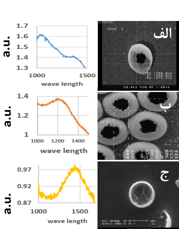
شکل ۳: تغییرات پیک طول موج با استفاده از تغییرات سایز دهانه ها. الف- سایز دهانه ۵۰۰ نانومتر- طول موج تحریک ۱۰۰۰ نانومتر. ب- سایز دهانه ۷۵۰ نانومتر- طول موج تحریک ۱۲۰۰ نانومتر. ج- سایز دهانه ۱۰۰۰ نانومتر- طول موج تحریک ۱۴۵۰ نانومتر.
