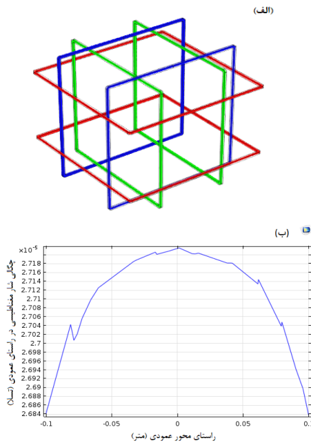
شکل ۲- شبیه سازی سه جفت پیچه هلمهولتز برای تولید میدان مغناطیسی در مرکز مجموعه (الف) و توزیع میدان مغناطیسی در مرکز پیچه ها برای یکی از سه جفت پیچه های هلمهولتز (ب).
