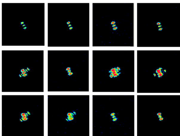
شکل ۴: نظیر شکل ۳ برای نوارهای دیود نور گسیل LB1 و LB4. نمایه های مدی IG_{2,2} و IG_{6,4} با تقارن زوج در تصاویر مشاهده می شود.
