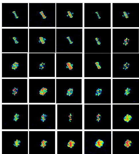
شکل ۶: نظیر شکل ۵ برای نوارهای دیود نور گسیل LB1، LB2 و LB3 و نمایه های گوناگون مدی (به متن مراجعه شود).
