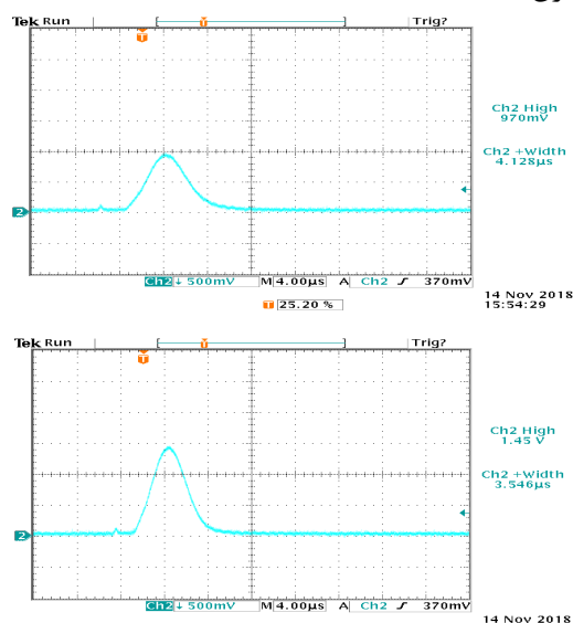
شکل ۴: نمونه هایی از رفتار زمانی جریان تخلیه برای مدار با ۴ لامپ درخش سری. ولتاژ شارژ خازن: بالا) ۱/۴ کیلو ولت، پایین) ۱/۸ کیلو ولت. پهنای زمانی تپ جریان به ترتیب ۴/۱۳ و ۳/۵۴ میکروثانیه و قله جریان تخلیه لامپ ۹۷ و ۱۴۵ آمپر است.
