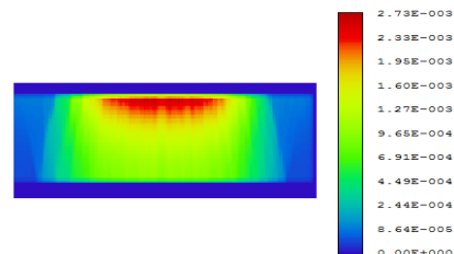
شکل ۴: پروفایل جذب در سطح مقطع تیغه با روزنه دمش.
