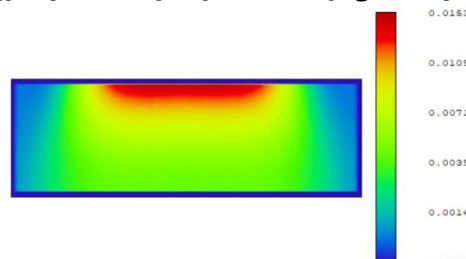
شکل ۹: پروفایل جذب در تیغه در دمش با استفاده از میکروعدسی.
