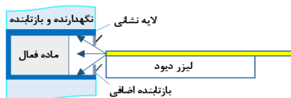
شکل ۳: طرحی از تیغه لیزر با لایه‌نشانی از سه طرف و روزنه دمش.
