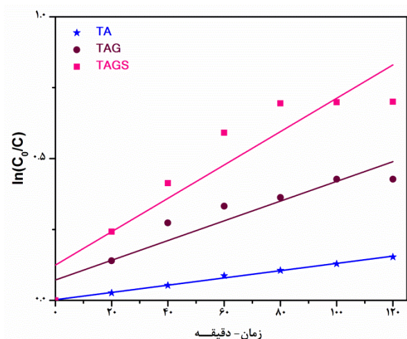
شکل ۲: نمودار ضریب k_{app} ایزوژل تیتانیا و نانوکامپوزیت‌های تولید شده.
