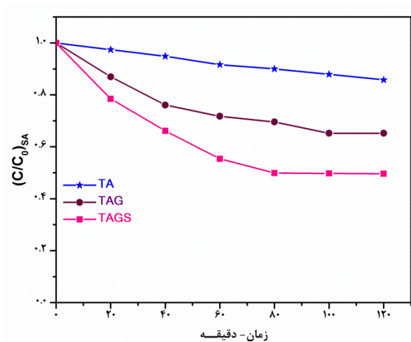
شکل ۱: نمودار غلظت نسبی ایزوژل تیتانیا و نانوکامپوزیت‌های تولید شده.
