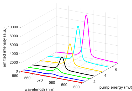
شکل ۳: طیف تابشی بر حسب طول موج متناظر با انرژی‌های دمش مختلف.
