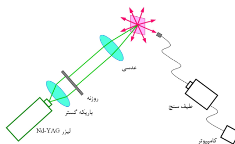
شکل ۲: طرح‌واره‌ی از چیدمان آزمایش.
