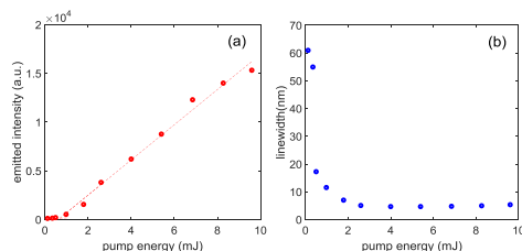
شکل ۳: (a) منحنی شدت بیشینه‌ی قله‌ی تابشی و (b) پهنا‌ی قله‌ی تابشی بر حسب انرژی هر پالس دمش.
