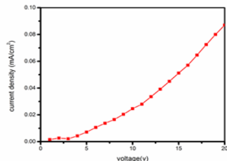
شکل ۶: نمودار ولتاژ-چگالی جریان دیود ساخته شده
