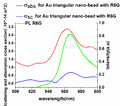
شکل ۷: منحنی سطح مقطع پراکندگی (آبی) و جذب (قرمز) برای بلور فوتونیک و طیف فلورئورسانس رودامین 6G (سبز)
