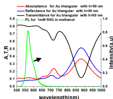
شکل ۶: منحنی طیف جذب (قرمز) و تراگسیل (سیاه) و بازتاب (آبی) برای بلور فوتونی و طیف فلورئورسانس رودامین- 6G (سبز).
