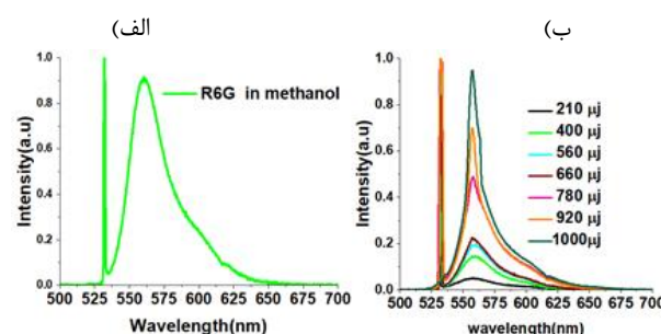
شکل ۳: (الف) طیف فلورسانس 1\text{mM} رودامین 6G در متانول روی زیر لایه سیلیکون (ب) طیف گسیلی لیزر پلاسمونی برای انرژی‌های دمش مختلف برای بلور فوتونیک ساخته شده از ذرات 382\text{nm} نانومتری پلی استایرن. خط تیز در 532\text{nm} مربوط به پرتو لیزر دمش می‌باشد.
