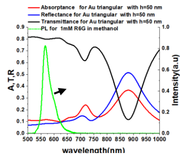
شکل ۶: منحنی طیف جذب (قرمز) و تراگسیل (سیاه) و بازتاب (آبی) برای بلور فوتونی و طیف فلئورسانس رودامین- 6G (سبز).
