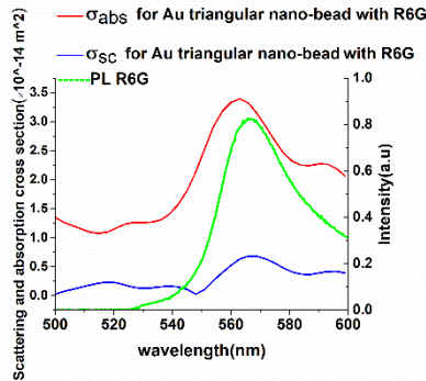
شکل ۷: منحنی سطح مقطع پراکندگی (آبی) و جذب (قرمز) برای بلور فوتونیک و طیف فلئورسانس رودامین 6G (سبز)
