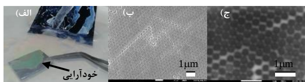
شکل ۱: (الف) خودآرایی ذرات پلی استایرن به قطر ۳۸۲ نانومتر روی سطح آب (ب) تصویر FE-SEM خودآرایی روی زیر لایه سیلیکون (ج) ساخت بلور فوتونیکی فلزی با شبکه هگزاگونال
