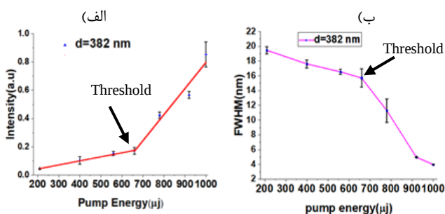
شکل ۴: (الف) منحنی شدت و (ب) پهنای در نصف بیشینه بر حسب انرژی دمش برای بلور فوتونی ساخته شده از ذرات به قطر 382\text{nm} نانومتر
