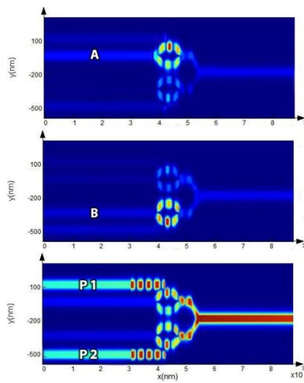
شکل ۵: توزیع میدان گیت منطقی پیشنهادی AND در حالات به ترتیب از بالا به پایین (۱) A=1, B=0 (۲) A=0, B=1 (۳) A=1, B=1
