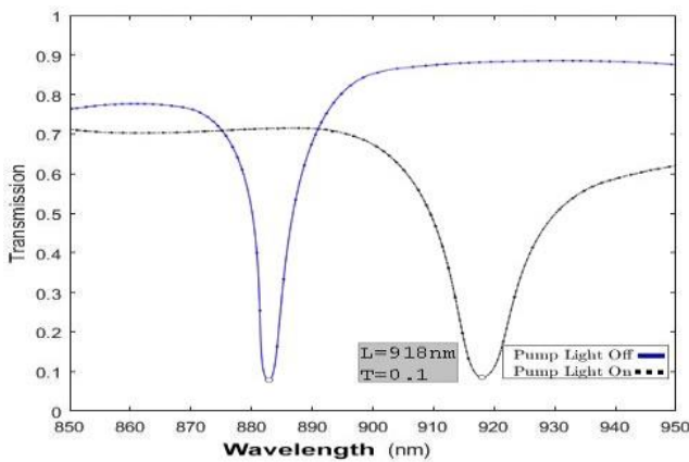
شکل ۳: شیفت طول موج قطع MZI.
