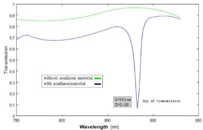
شکل ۲: میزان عبوردهی MZI بر حسب طول موج در حضور و عدم حضور بازوی غیرخطی.
