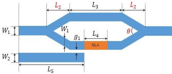
شکل ۱: تصویر شماتیک از ساختار پایه یک سیستم سوئیچینگ تمام نوری مبتنی بر MZI.
