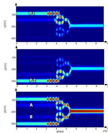
شکل ۴: توزیع میدان گیت منطقی پیشنهادی OR در حالات به ترتیب از بالا به پایین (۱) A=1, B=0 (۲) A=0, B=1 (۳) A=1, B=1
